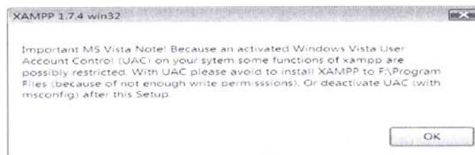
Gambar 5.1 Permission XAMPP
