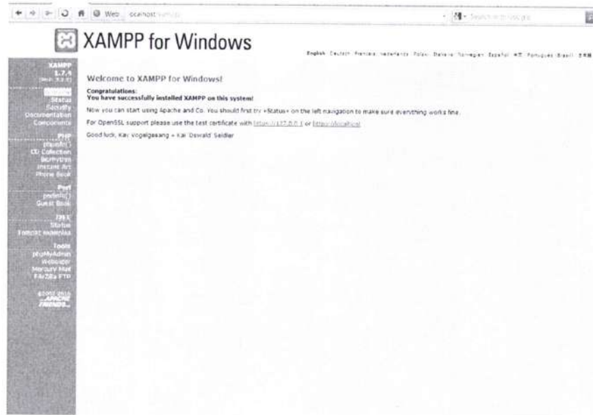
Gambar 5.5 Halaman XAMPP
